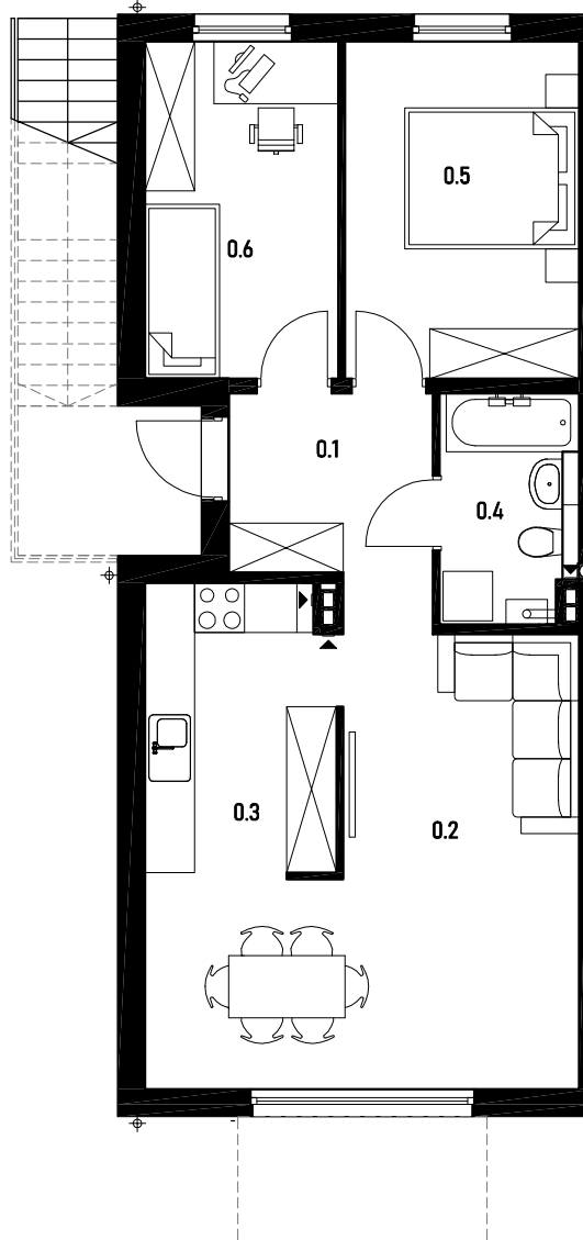
rzut kondygnacji 1:100
