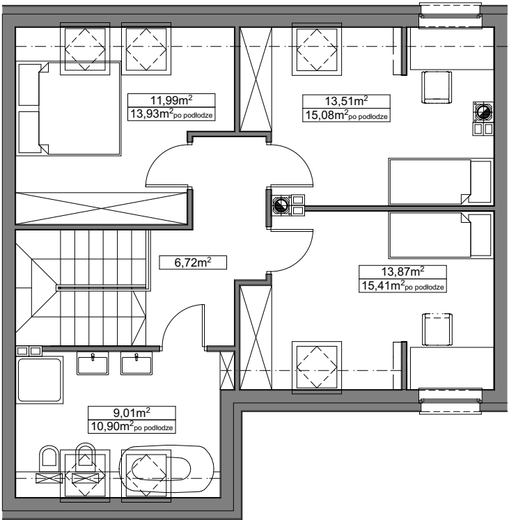
poddasze, skala 1:100
