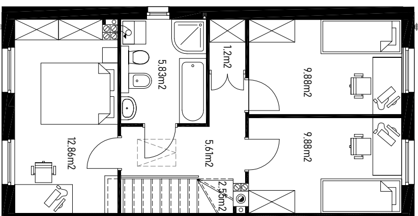
piętro 1:100
