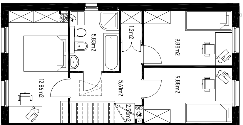
piętro 1:100
